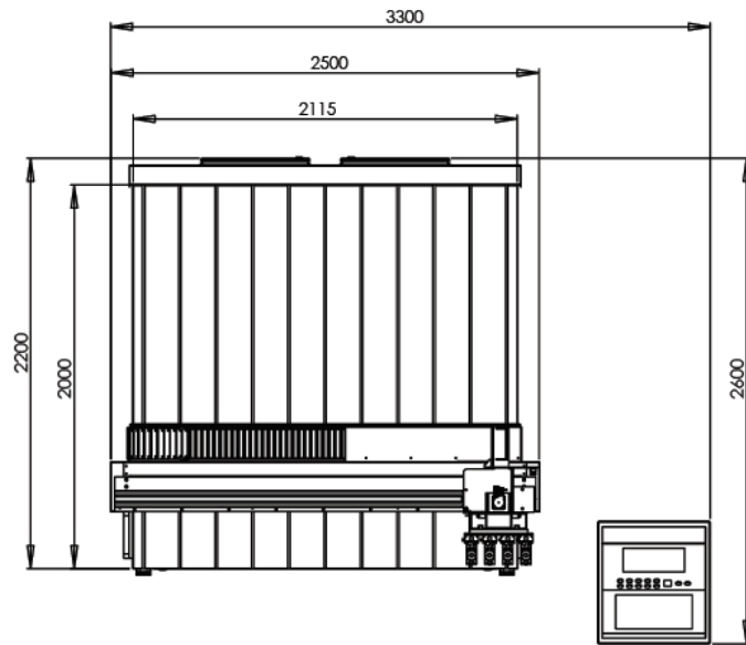
Felülnézet
