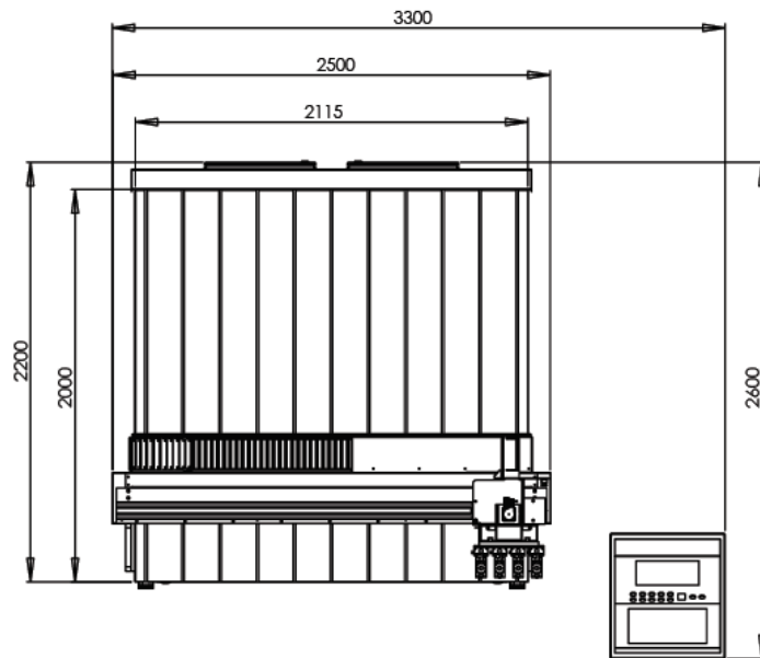
Szemből nézet
